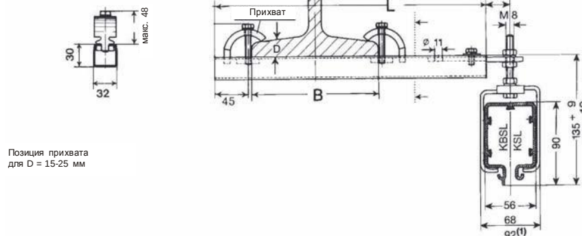
Сечение без кронштейна
